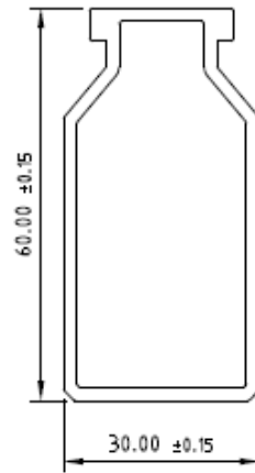
Fin Profile 30 x 60 mm
