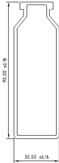
Fin Profile 30 x 90 mm
